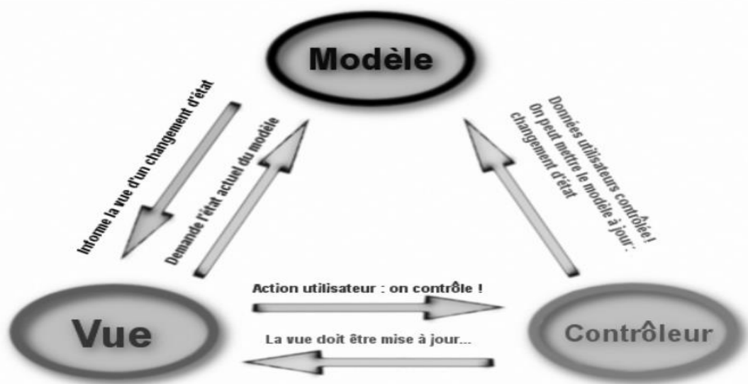
Figure 12: Modèle MVC
