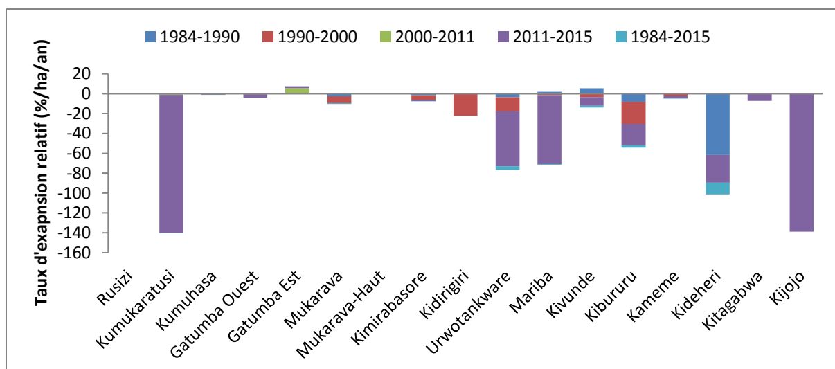
Figure 48: Taux relatifs d'expansion spatiale des plans d'eau de 1984 à 2015
