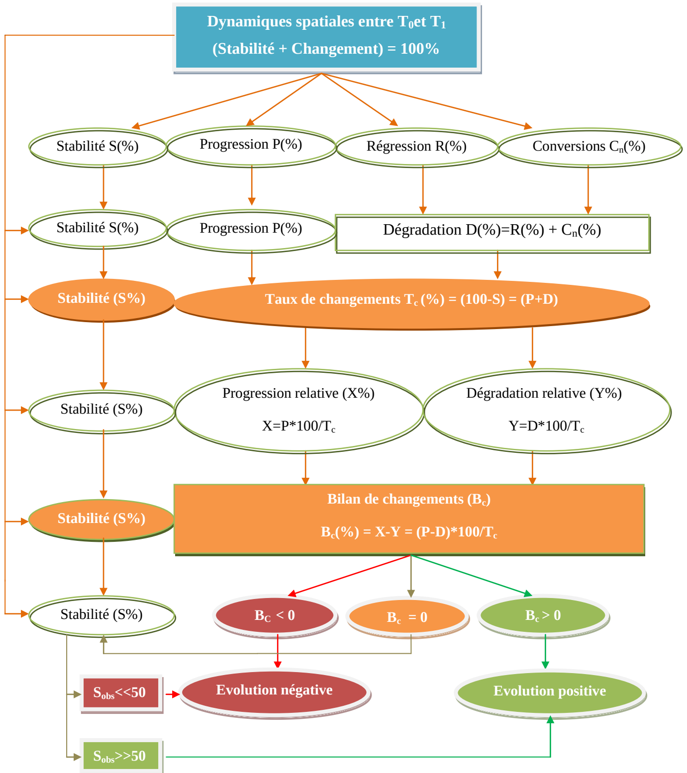
Figure 18: Algorithme de détermination des indices de tendance (Auteur, 2017)
