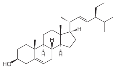
Stigmastérol
