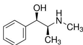
Ephédrine
