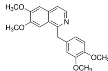
Papavérine
