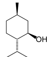
Menthol
