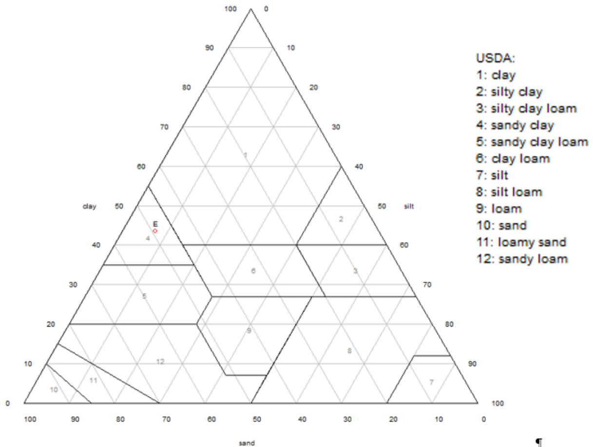
Figure 3 : Représentation du sol du site d'essai (E) sur le triangle texturale du USDA
