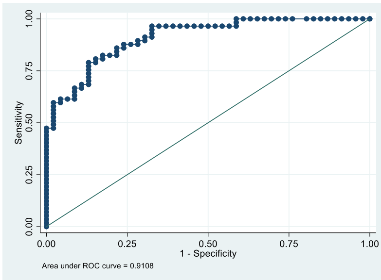
Figure 5 : La courbe ROC(AUC)
