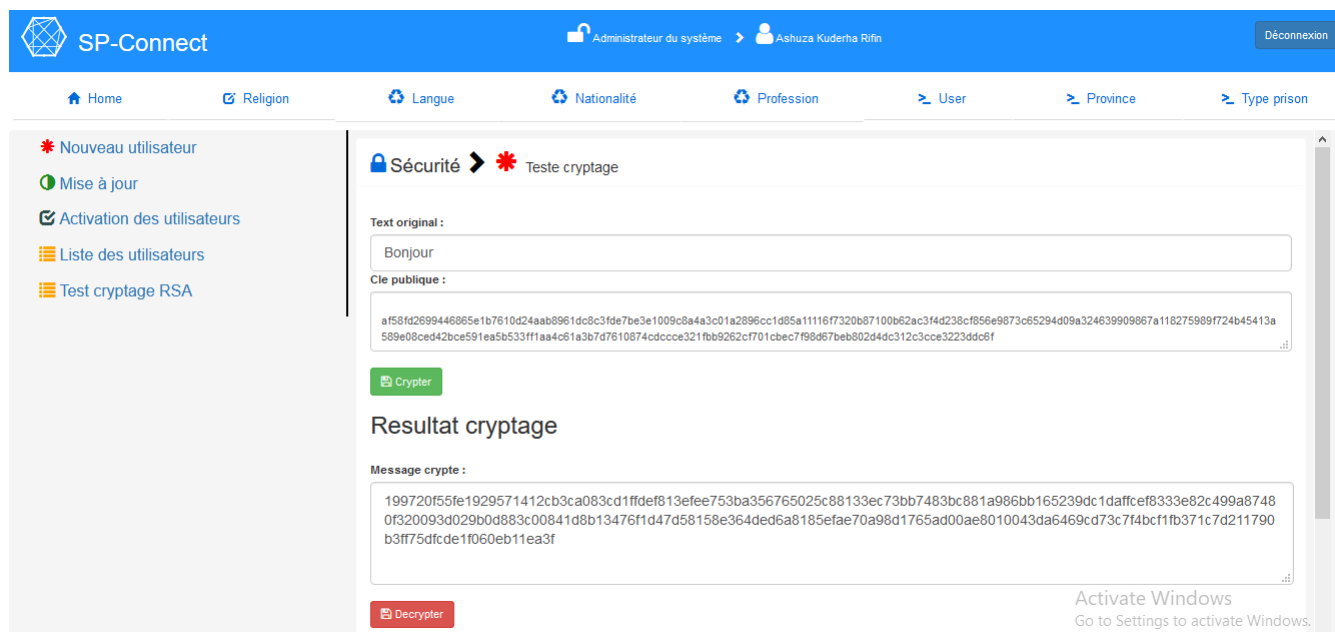
FIGURE 5.2 – Résultat du cryptage
