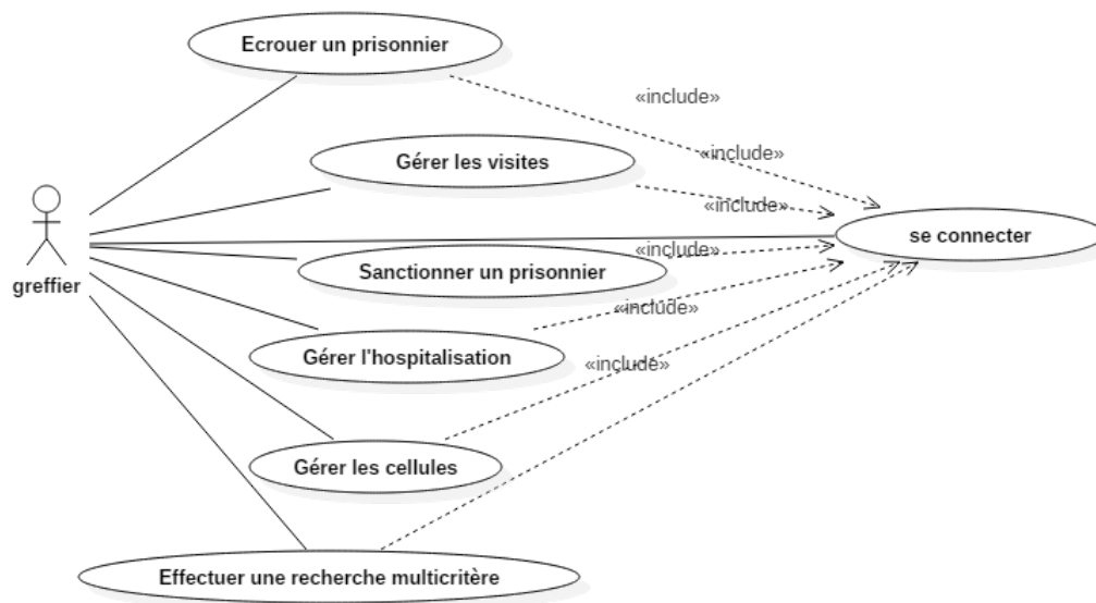
FIGURE 3.2 – Cas d'utilisation «Effectuer les opérations pénitentiaires»
