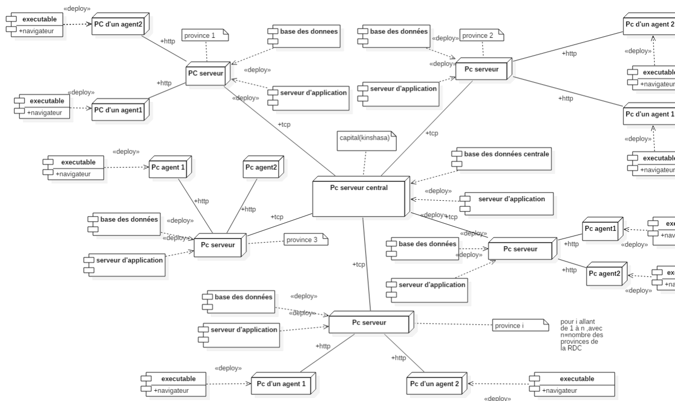
FIGURE 3.9 – Diagramme de déploiement en local
