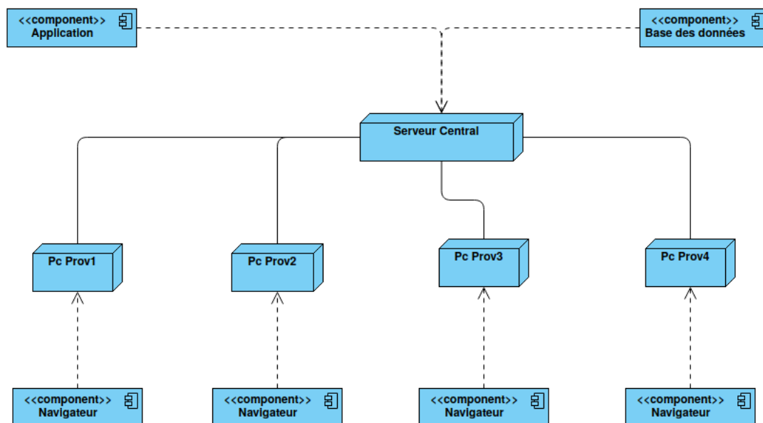
FIGURE 3.10 – Diagramme de déploiement en ligne
