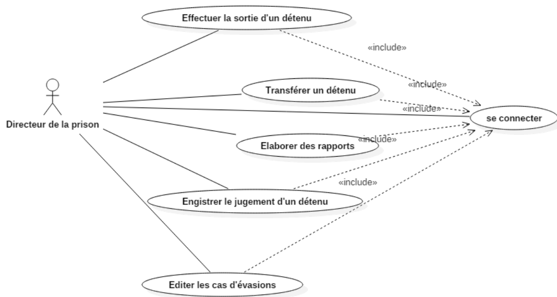
FIGURE 3.3 – Cas d'utilisation «Gérer le dossier administratif du détenu»
