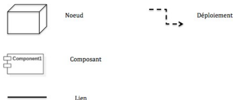
FIGURE 3.8 – symboles utilisés dans la construction du diagramme de déploiement
