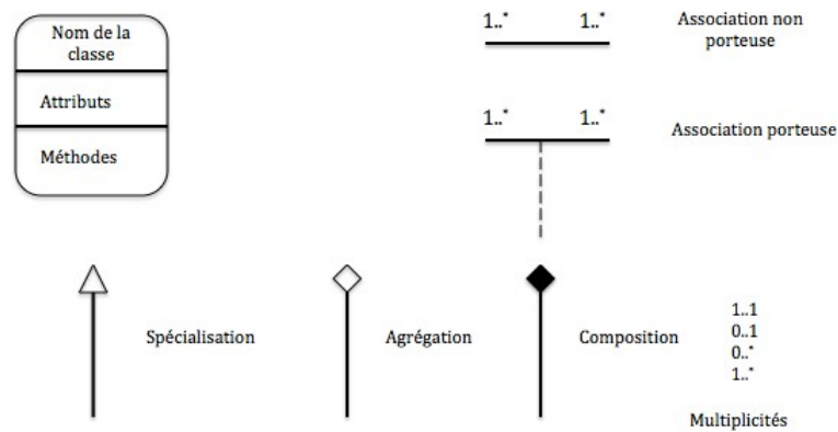
FIGURE 3.6 – symboles utilisés dans la construction du diagramme des classes
