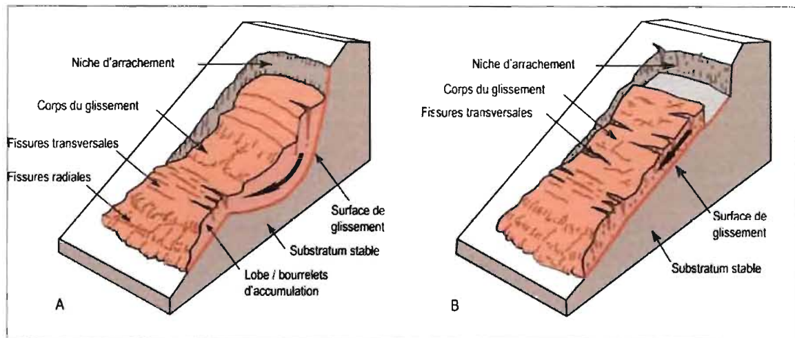
Figure 25 : Types de glissements de terrain
