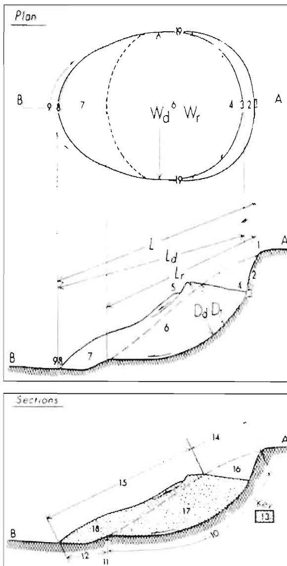
Figure 24 : Description des éléments morphométriques et morphologiques composant un glissement terrain
