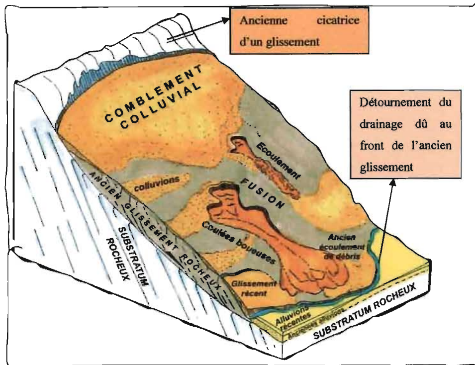
Figure 28 : Mouvement complexe de type glissement-coulé
