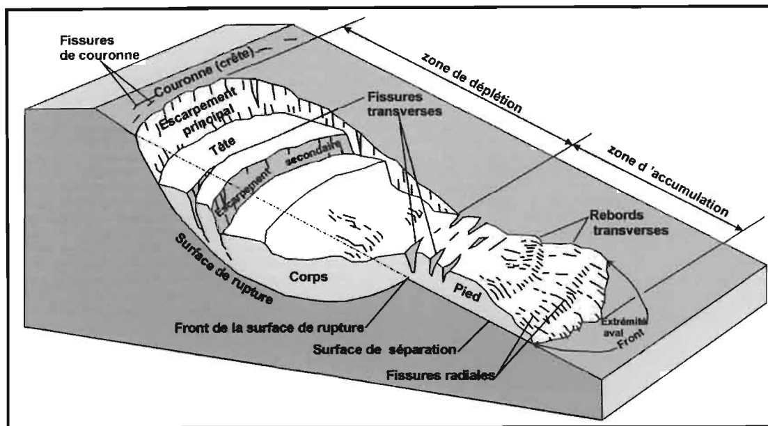
Figure 23 : Bloc diagramme d'un glissement de terrain idéal
