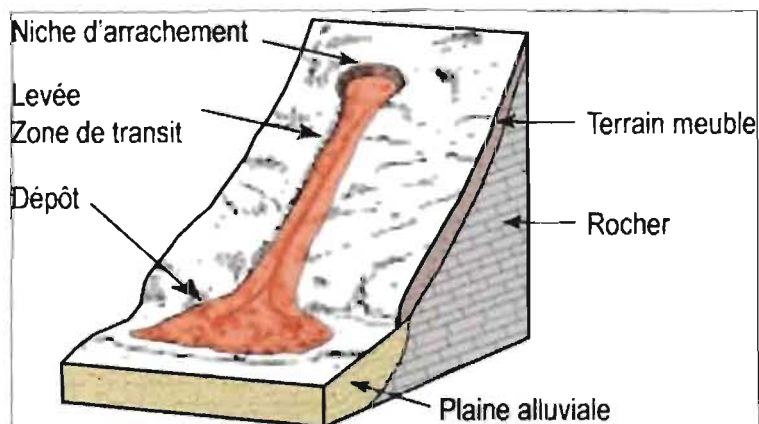
Figure 26 : Coulée de boues
