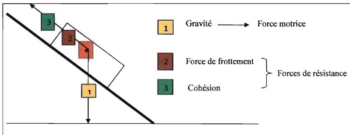
Figure 21 : Rapport de forces pour les conditions de glissement
