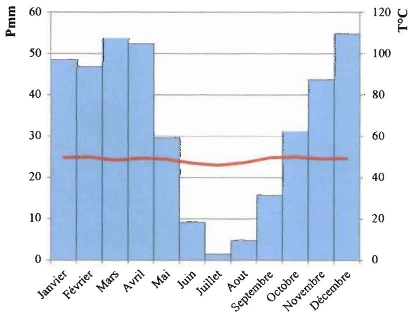
Figure 7 : Diagramme ombrothermique à la station de Bujumbura-Aéroport
