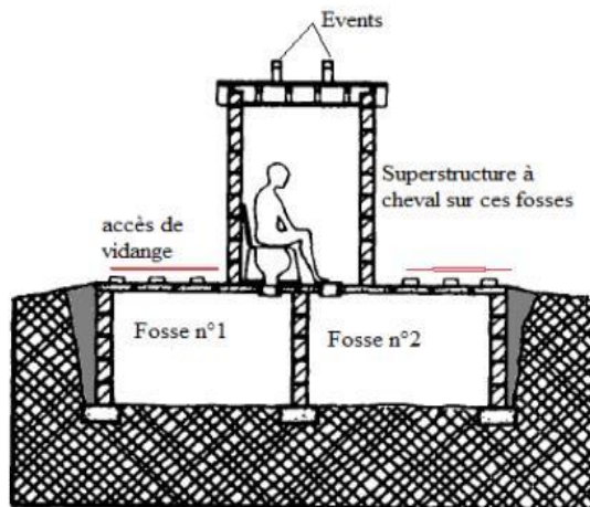
Latrine VIP à double fosse (Kalbermatten et al. , 1980)
