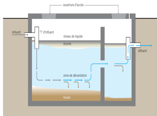
Schéma d'une fosse septique (Tilley et al. , 2008)
