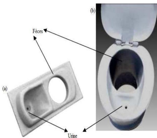
Latrine avec déviation d'urine (a), cuvette de toilette (b) (Langergraber & Muellegger, 2005)
