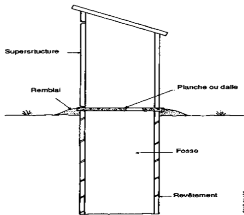
Schéma d'une latrine à simple fosse (Franceys et al. , 1995)
